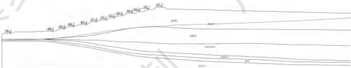
图 5.1-10 827.5m 滩顶标高南侧坝体洪水工况浸润线图
